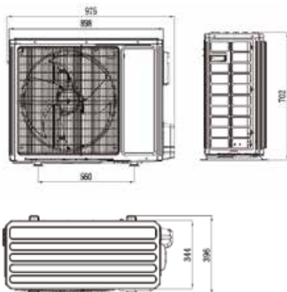
Wymiary jednostki zewnętrznej split IGZAW6SNO-1
