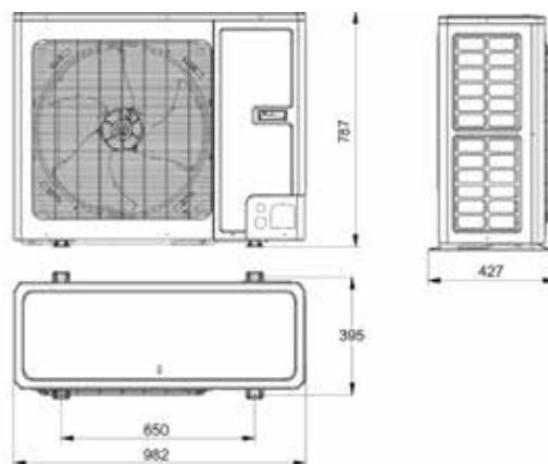
Wymiary jednostki zewnętrznej split IGZAW8SNO-1, IGZAW10SNO-1, IGZAW8SNO3-1, IGZAW10SNO3-1
