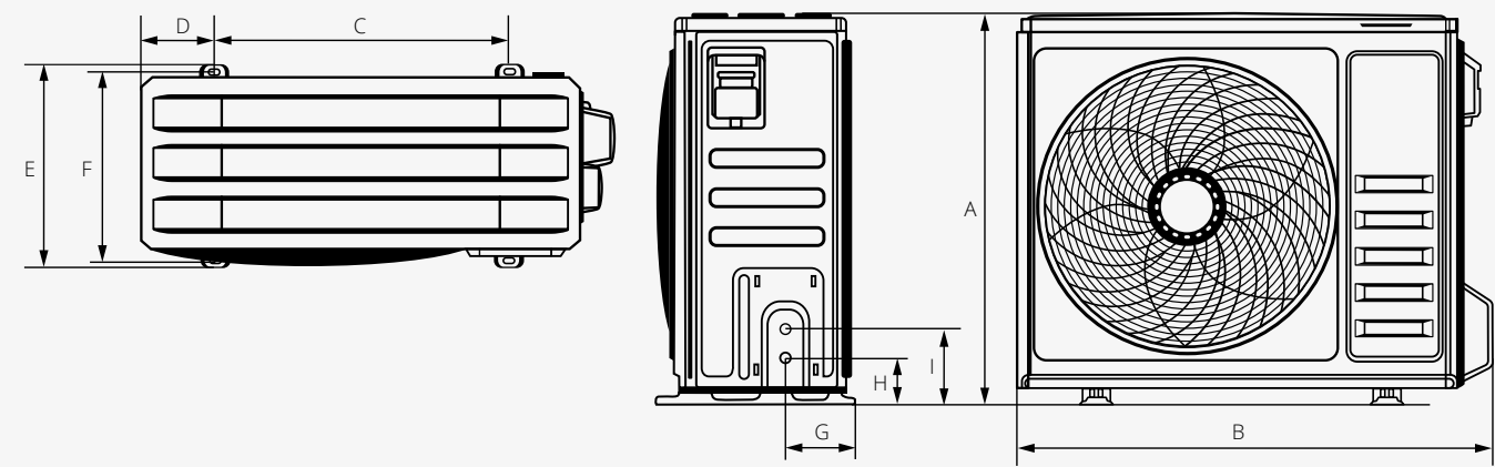
Jednostka zewnętrzna 4/6/8/10 kW Rotenso Heatmi Split
