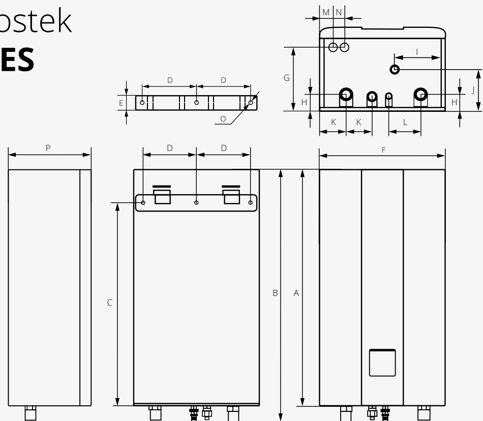
Jednostka wewnętrzna 6/8/10 kW Rotenso Heatmi Split
