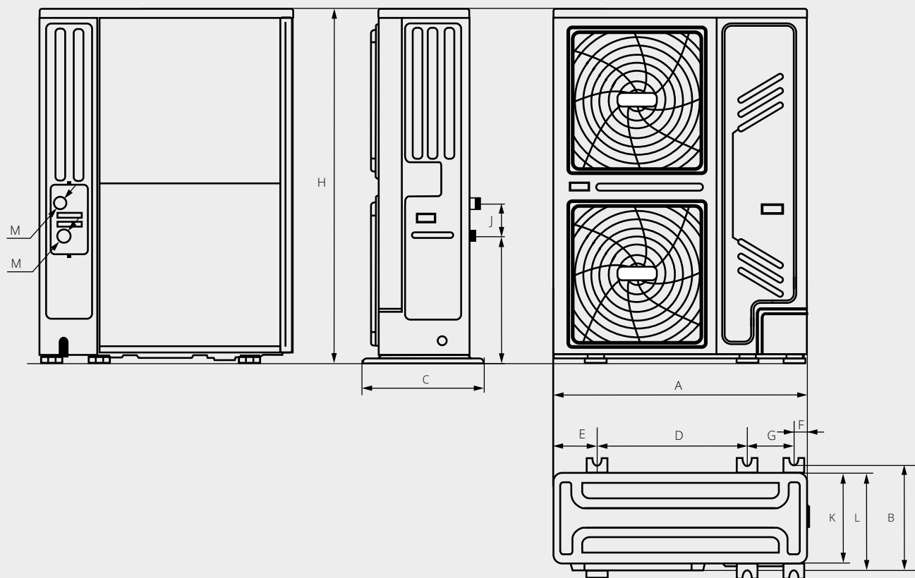
Jednostka zewnętrzna 22/30 kW Rotenso Aquami Big Mono
